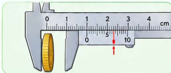
Gambar 2. Hasil pengukuran tebal sebuah koin logam
