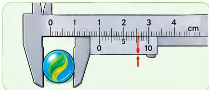
Gambar 1. Hasil pengukuran diameter sebuah kelereng
