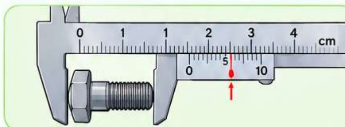
Gambar 5. Hasil pengukuran diameter sebuah baut
